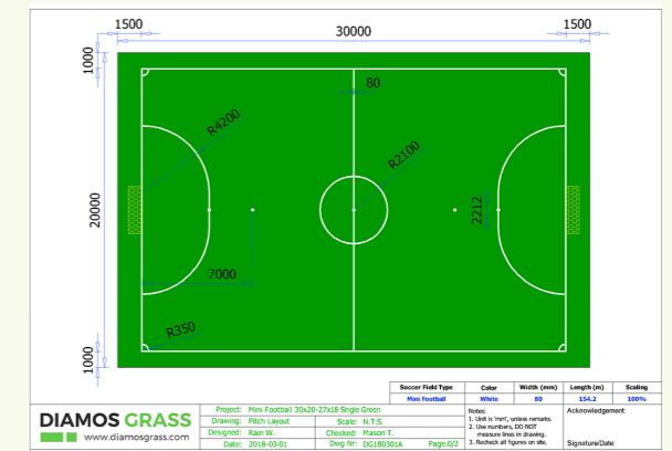
Mini Football 30x20-27x18 Single
